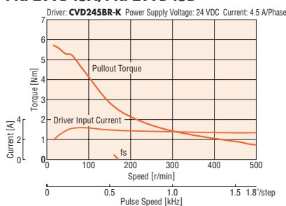
PKP299D63A/ PKP299D63B
