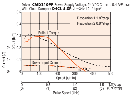
PKP244U04A/PKP244U04B
