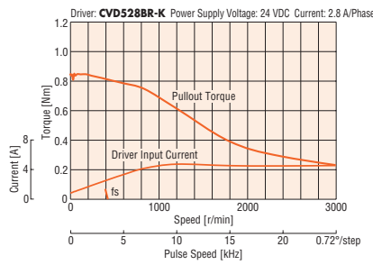
PKP566N28A2/PKP566N28B2
