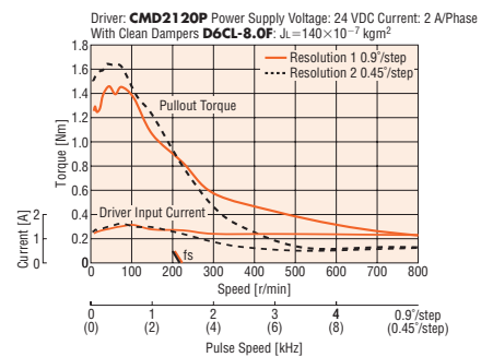
PKP268MU20A/PKP268MU20B
