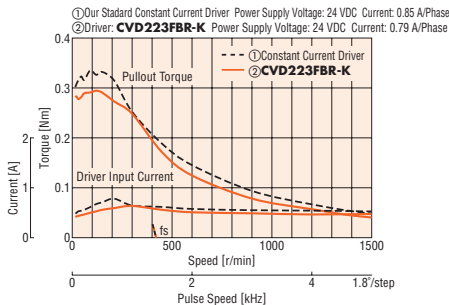
PKP244D08A2/ PKP244D08B2
