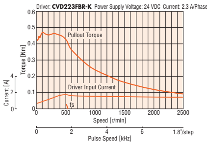
PKP244D23M2
